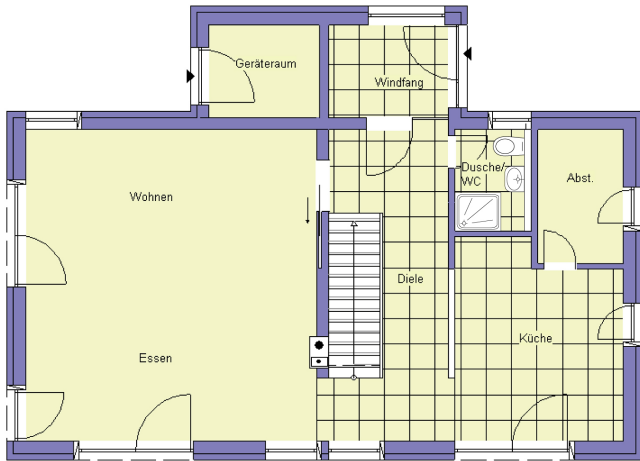
Erdgeschoss
