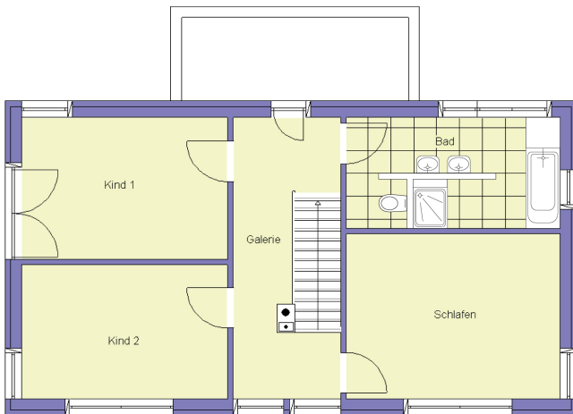
Dachgeschoss
