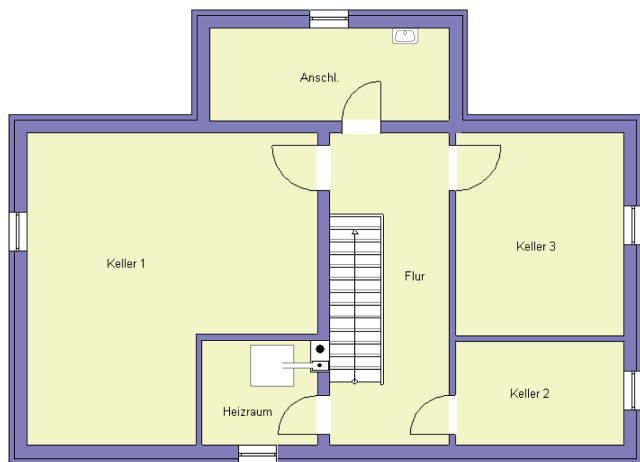
Kellergeschoss
