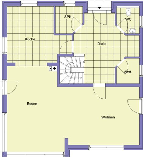
Erdgeschoss
