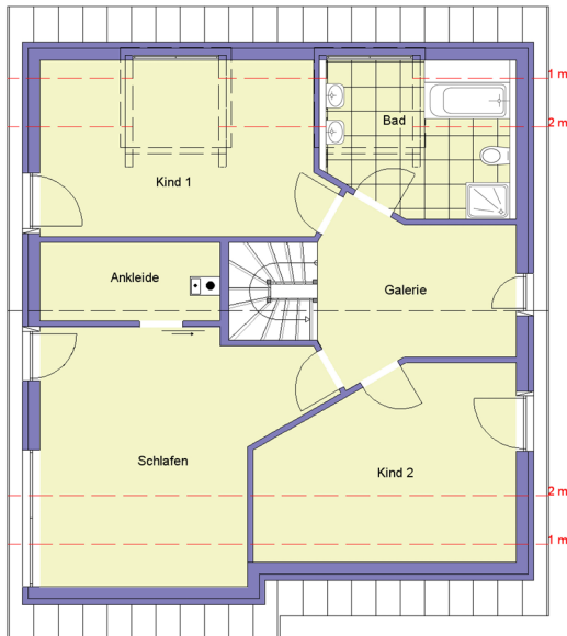
Dachgeschoss
